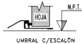
UMBRAL C/ESCALÓN
